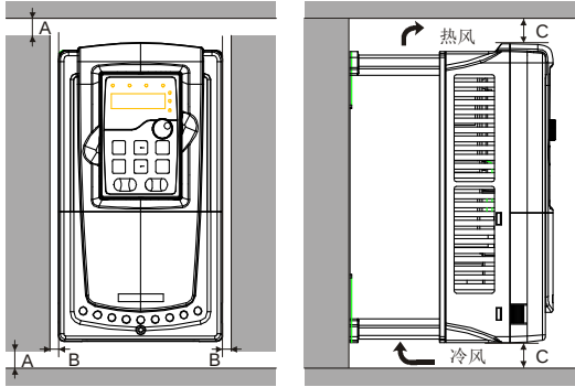
图 4-3 单台安装
