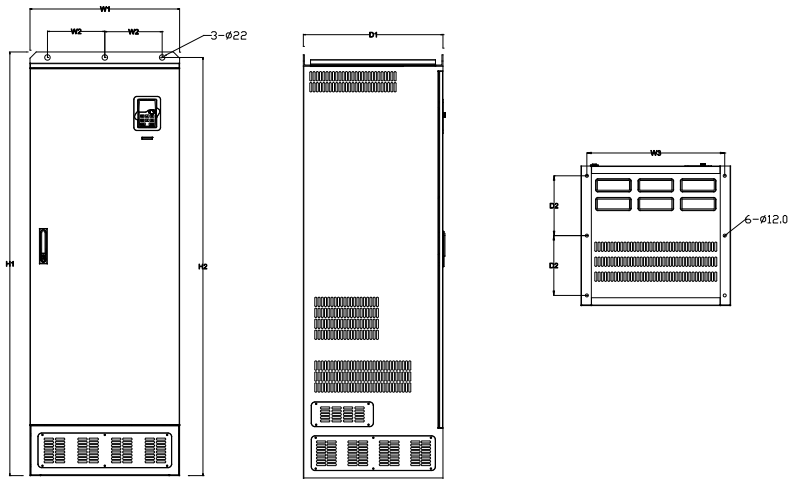
图 C-17 660V 400-630kW 落地安装
