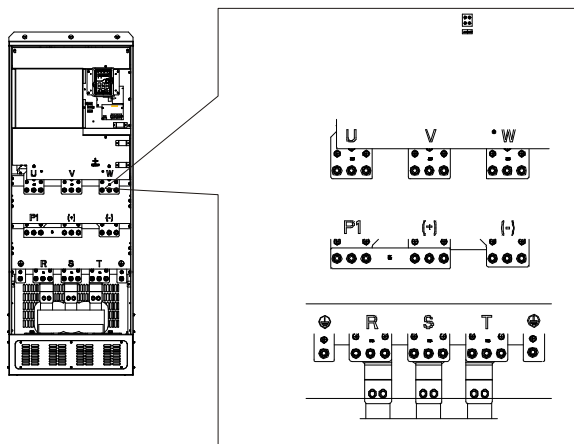
图 4-18 660V 400~630kW 主回路端子
