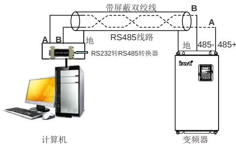
图 11-1 RS485 单机应用时的物理接线
