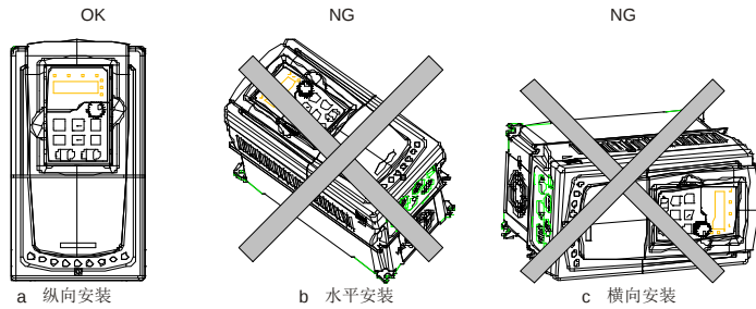
图 4-1 变频器安装方向
