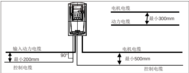
图 D-3 布线距离
