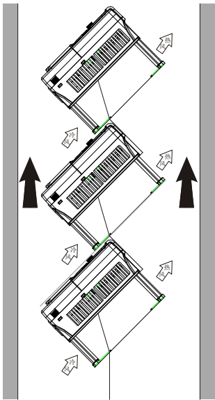
图 4-6 倾斜安装
