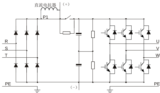
图 3-2 380V 37kW（含）以上主回路简图
