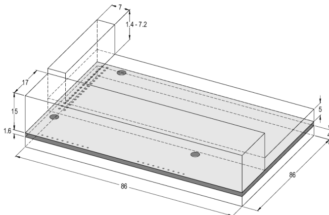
图 A-2 EC-TX103 通讯卡外形尺寸（单位：mm）
