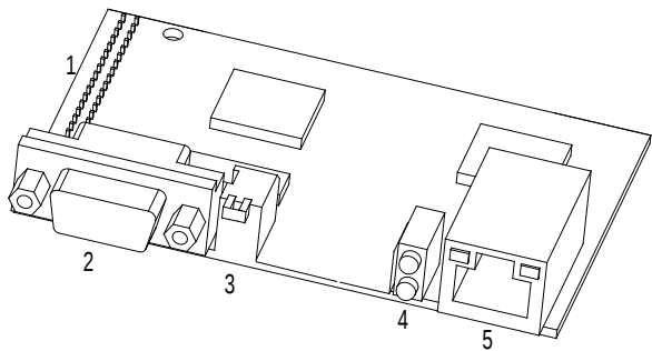
图 A-1 EC-TX1033 通讯卡外形
