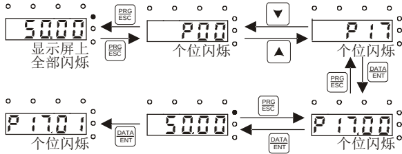
图 5-5 查看参数
