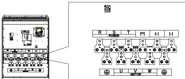
图 4-17 380V 220~315kW、660V 250~350kW 主回路端子
