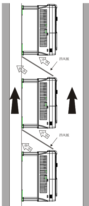
图 4-5 垂直安装
