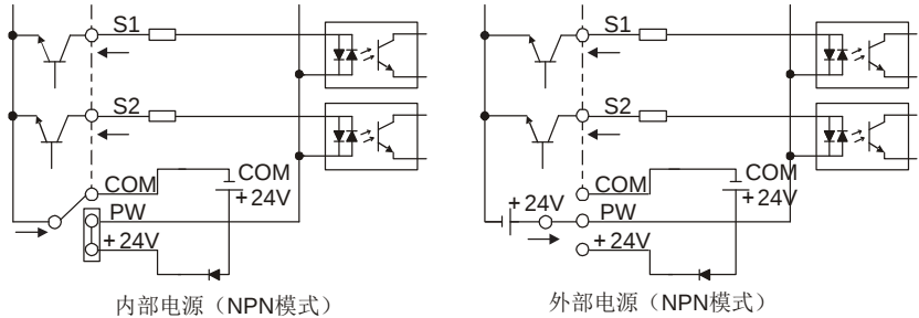
图 4-22 NPN 模式
