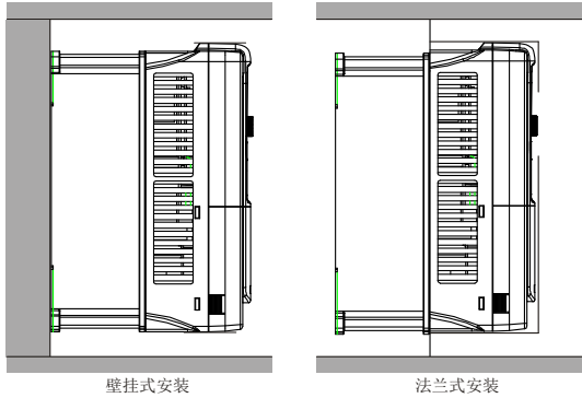
图 4-2 安装方式
