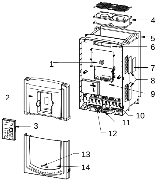
图 3-6 产品结构
