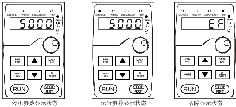
图 5-2 状态显示
