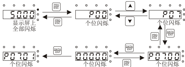
图 5-4 设定密码
