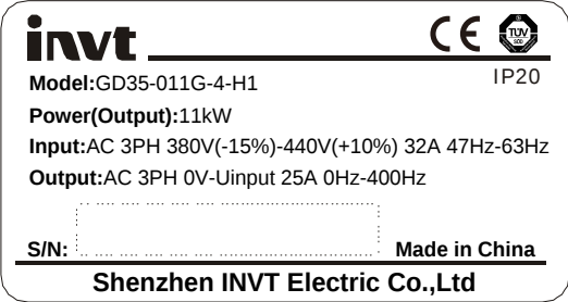
图 3-4 产品铭牌
