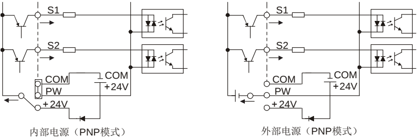
图 4-23 PNP 模式
