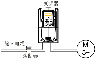
图 4-24 熔断器配置
