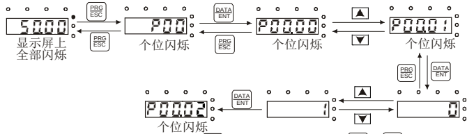
图 5-3 修改参数
