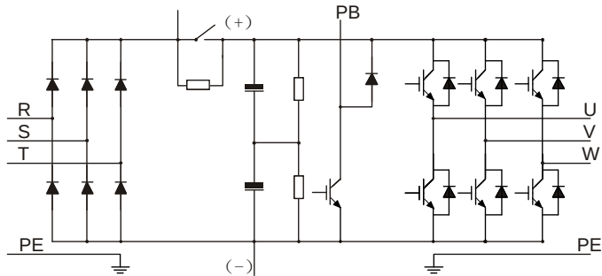
图 3-1 380V 30kW（含）以下主回路简图
