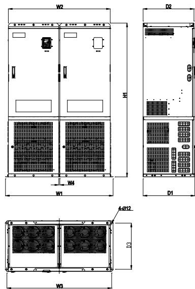
图 B-18 380V 710~3000kW 并机安装
