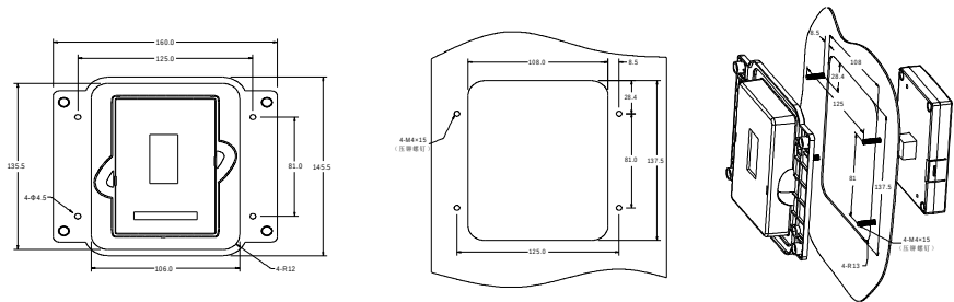
键盘转接支架
