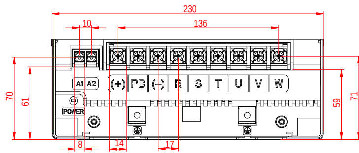
图 4-13 380V 018G/022P 主回路端子
