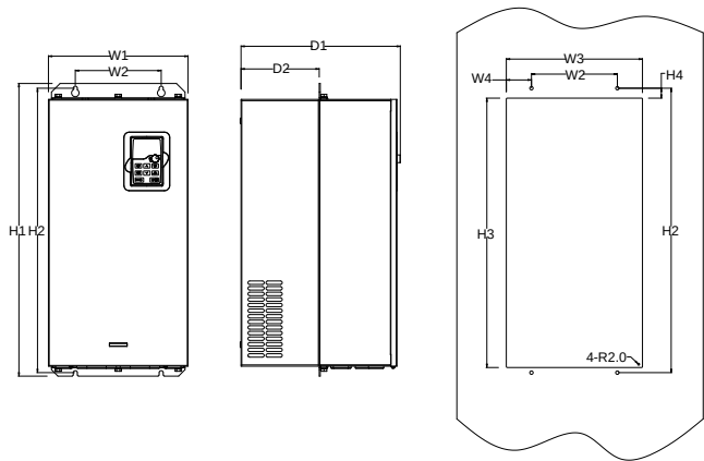
图 B-10 037G/045P~110G/132P 法兰安装
