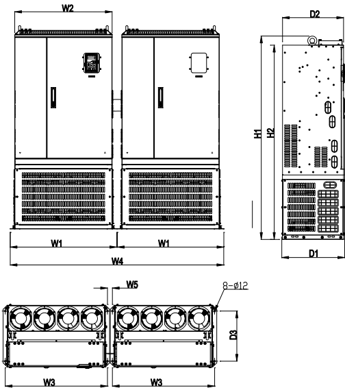
图 B-15 380V 560~630kW 并机安装
