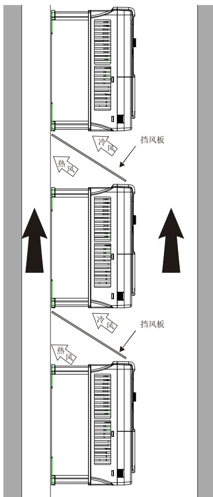
图 4-4 垂直安装
