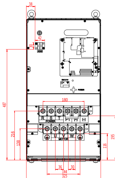
图 4-16 380V 075G/090P~110G/132P 主回路端子
