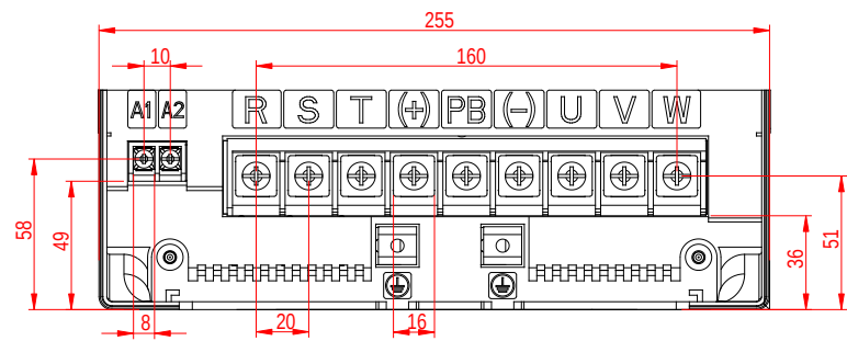
图 4-14 380V 022G/030P~030G/037P 主回路端子
