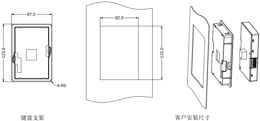
图 B-1 键盘安装架（选配）
