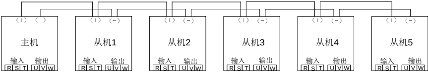
图 4-9 并机主回路接线
