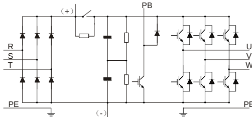
图 3-1 380V 030G/037P 及以下主回路
