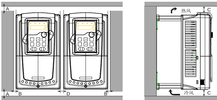
图 4-3 并行安装
