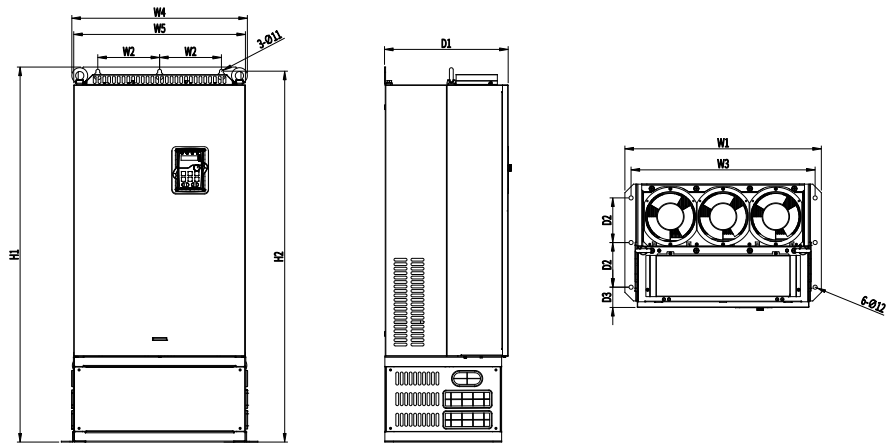
图 B-12 132G/160P~200G/220P 落地安装（带底座）
