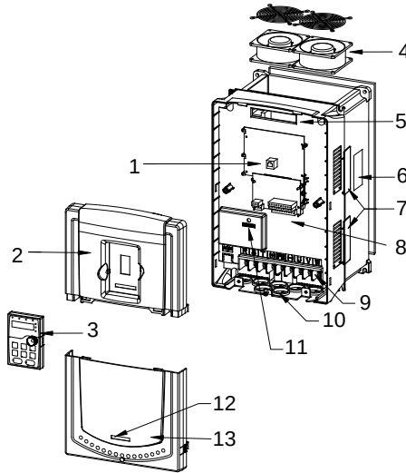
图 3-6 产品结构
