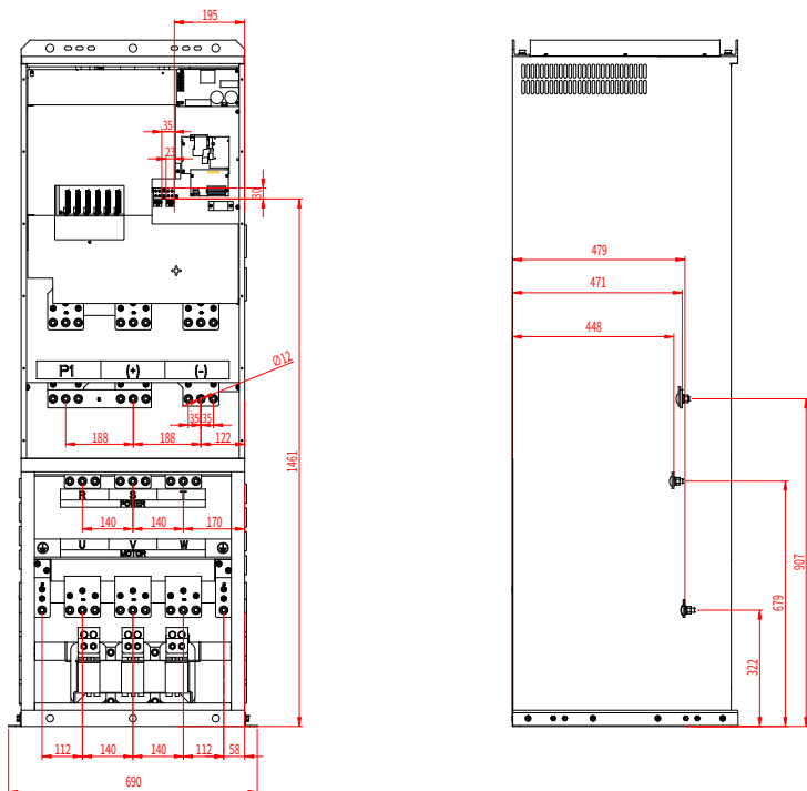
图 4-21 380V 710G~3000G 主回路端子
