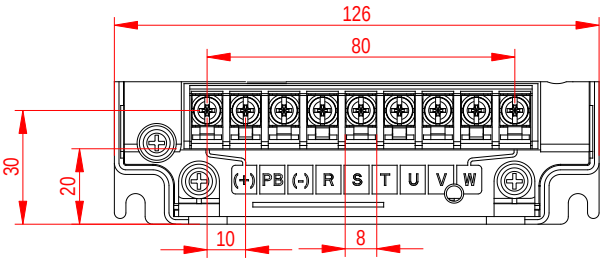
图 4-10 380V 0R7G-2R2G 主回路端子
