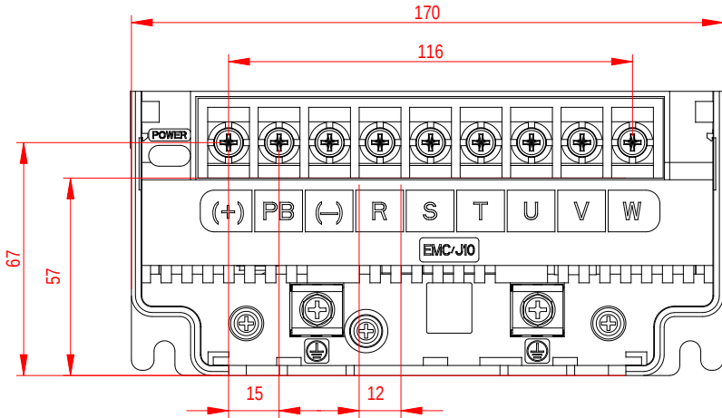
图 4-12 380V 7R5G/011P~015G/018P 主回路端子
