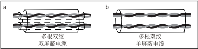
图 C-3 动力电缆布线
