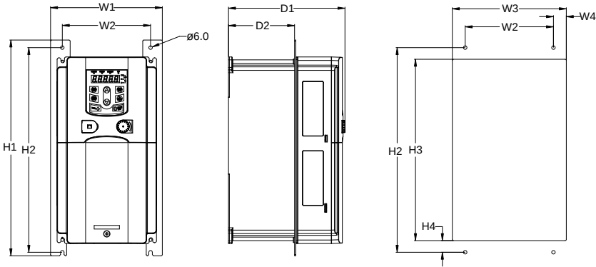
图 B-8 0R7G~015G/018P 法兰安装
