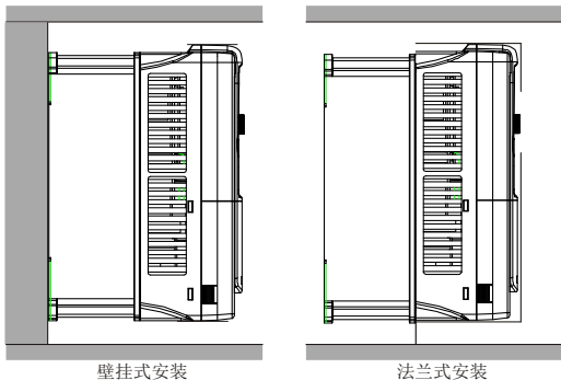
图 4-2 安装方式
