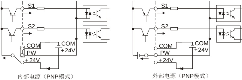
图 4-30 PNP 模式
