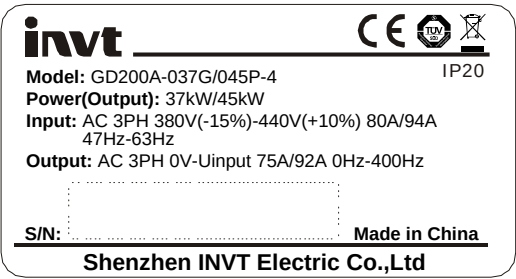
图 3-4 产品铭牌
