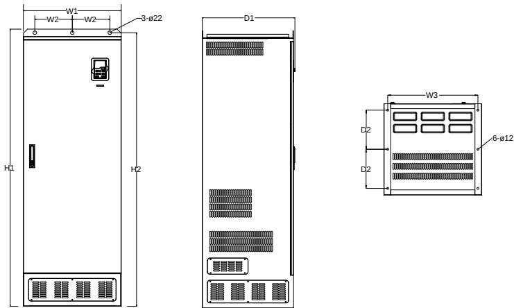
图 B-14 355G/400P~500G 落地安装
