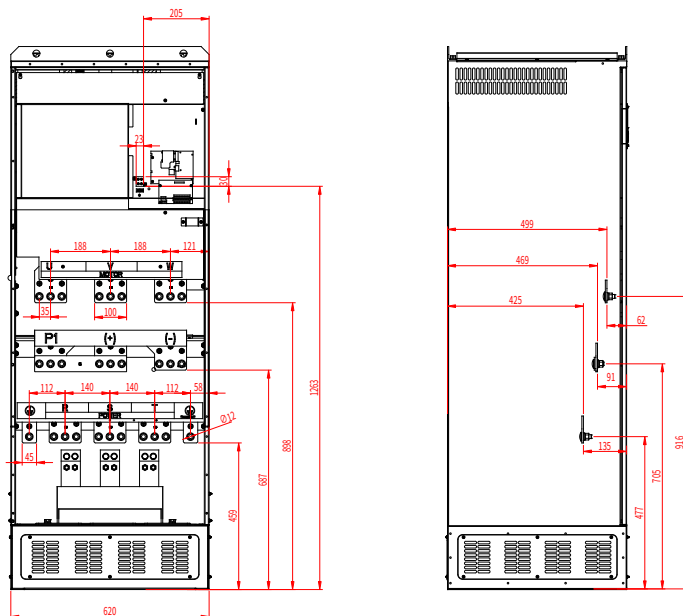
图 4-19 380V 355G/400P~500G 主回路端子
