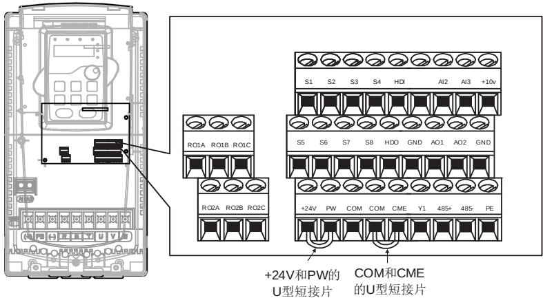
图 4-27 380V 015G/018P 及以下 U 型短接位置
