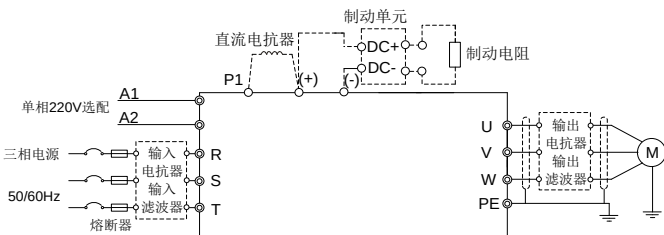
图 4-8 380V 037G/045P 及以上主回路接线
