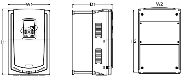
图 B-4 018G/022P~030G/037P 壁挂安装
