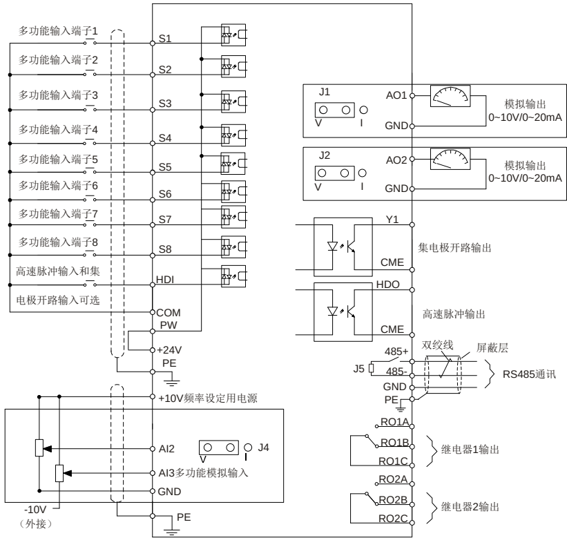
图 4-23 控制回路接线
