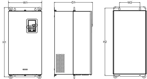
图 B-5 037G/045P~110G/132P 壁挂安装
