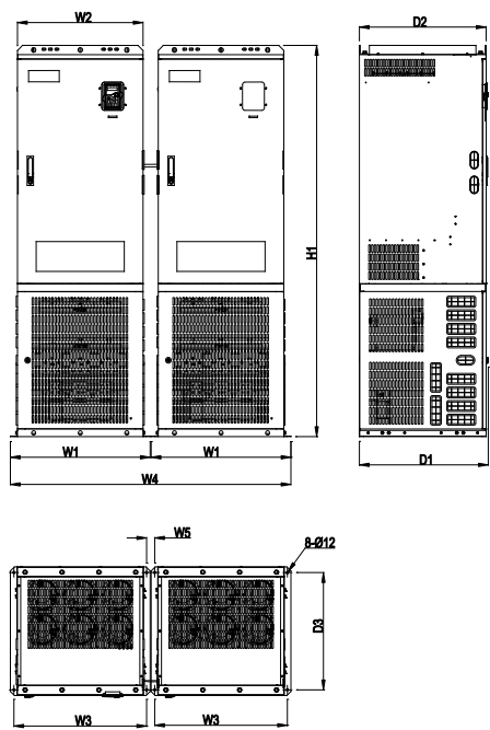
图 B-16 380V 710~3000kW 并机安装
