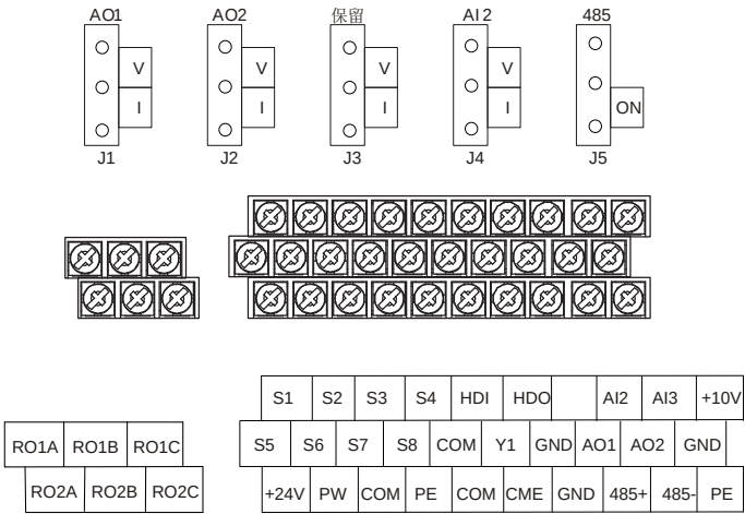
图 4-26 380V 018G/022P 及以上控制端子
