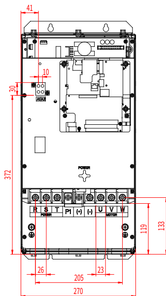
图 4-15 380V 037G/045P~055G/075P 主回路端子
