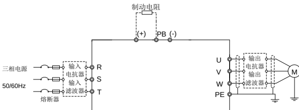
图 4-6 380V 5R5G/7R5P 及以下主回路接线
