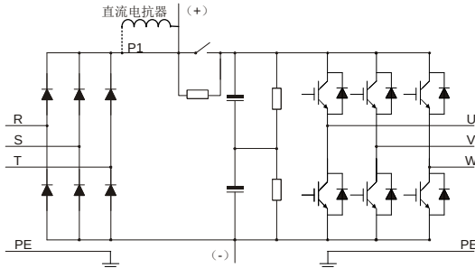
图 3-2 380V 037G/045P~315G/355P 主回路
