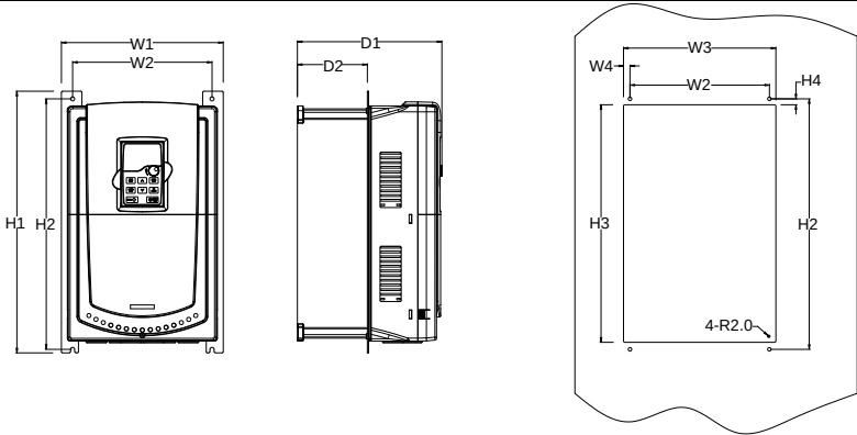
图 B-9 018G/022P~030G/037P 法兰安装
