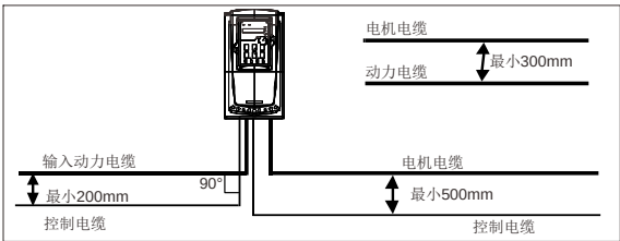
图 C-4 布线距离
