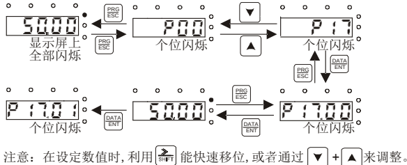
图 5-7 查看参数
