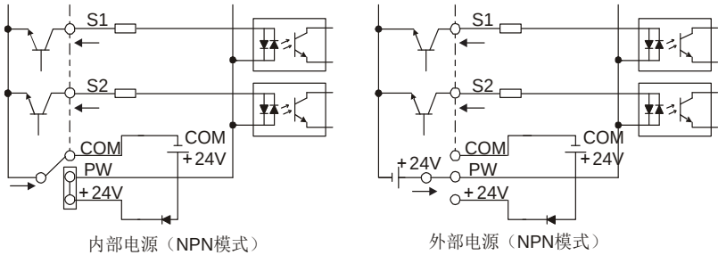
图 4-29 NPN 模式
