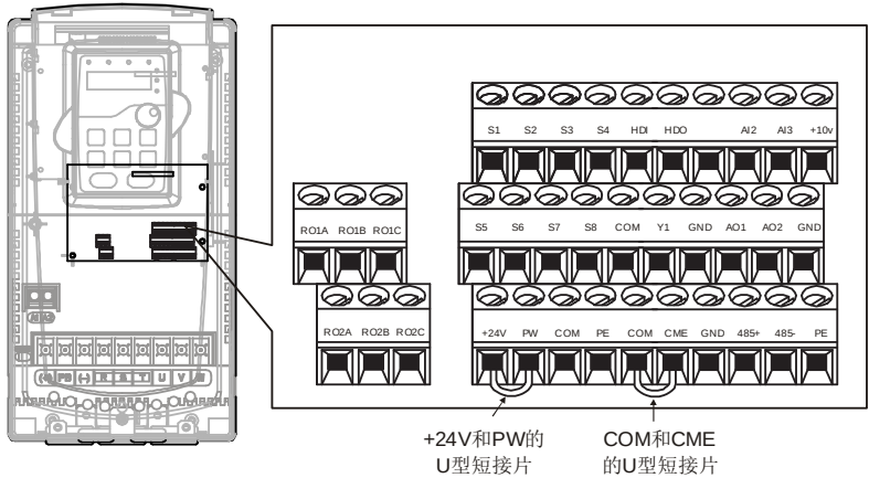
图 4-28 380V 018G/022P 及以上 U 型短接位置
