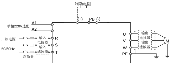
图 4-7 380V 7R5G/011P~030G/037P 主回路接线
