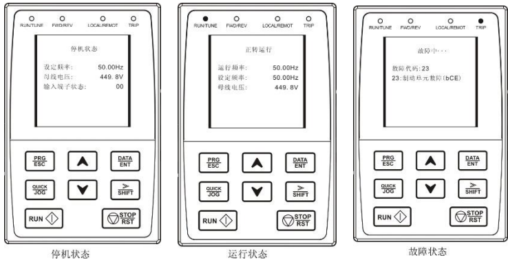
图 5-8 状态显示
