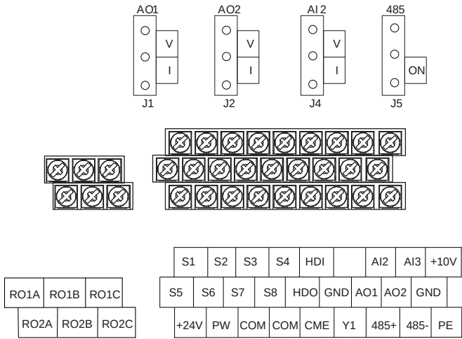
图 4-25 380V 015G/018P 及以下控制端子
