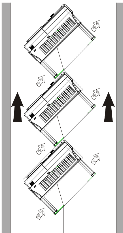
图 4-5 倾斜安装
