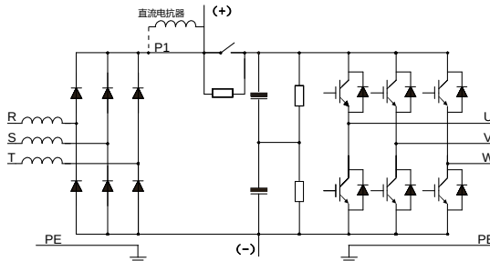
图 3-3 380V 355G/400P 及以上主回路
