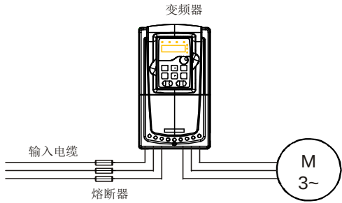
图 4-31 熔断器配置
