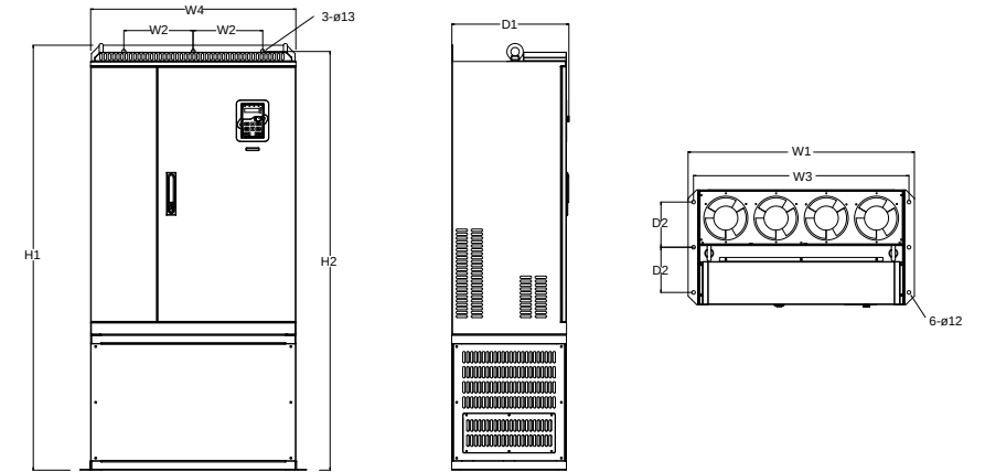
图 B-13 220G/250P~315G/355P 落地安装（带底座）
