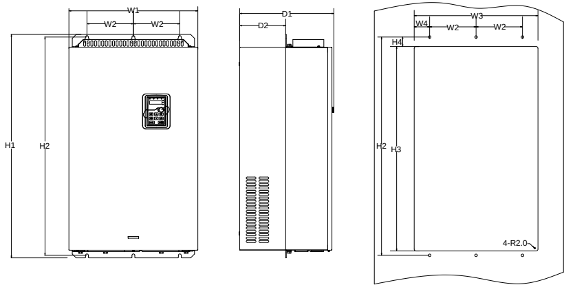
图 B-11 132G/160P~200G/220P 法兰安装
