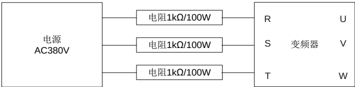
图 8-1 380V 驱动装置充电电路示例
