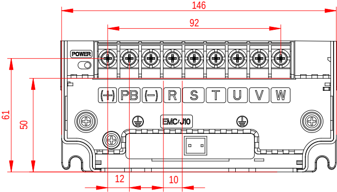
图 4-11 380V 004G/5R5P-5R5G/7R5P 主回路端子
