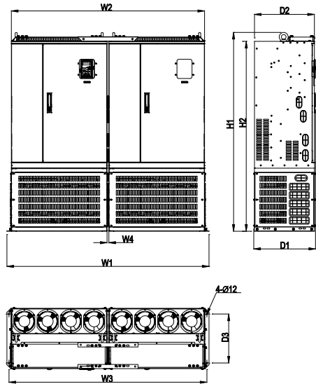
图 B-17 380V 560~630kW 并机安装
