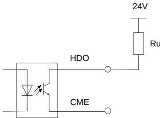
图 4-24 HDO 接线
