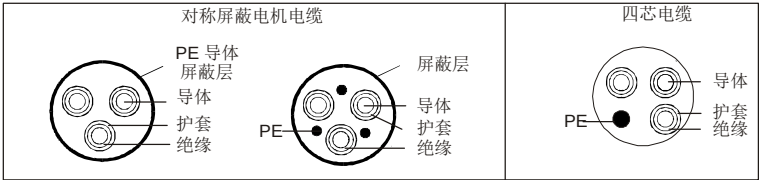
图 C-1 对称屏蔽电机电缆
