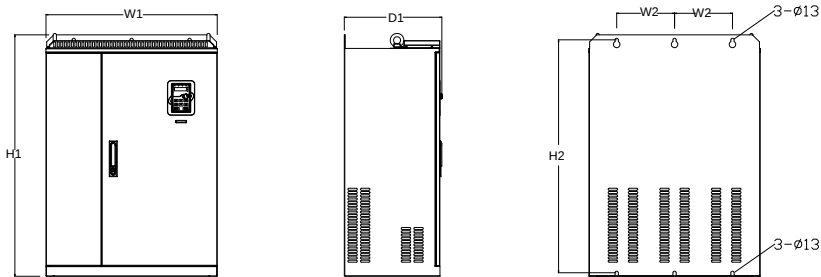
图 B-7 220G/250P~315G/355P 壁挂安装
