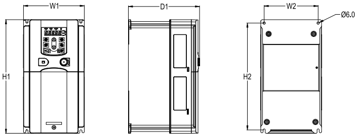
图 B-3 0R7G~015G/018P 壁挂安装
