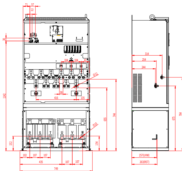
图 4-20 380V 560G~630G 主回路端子
