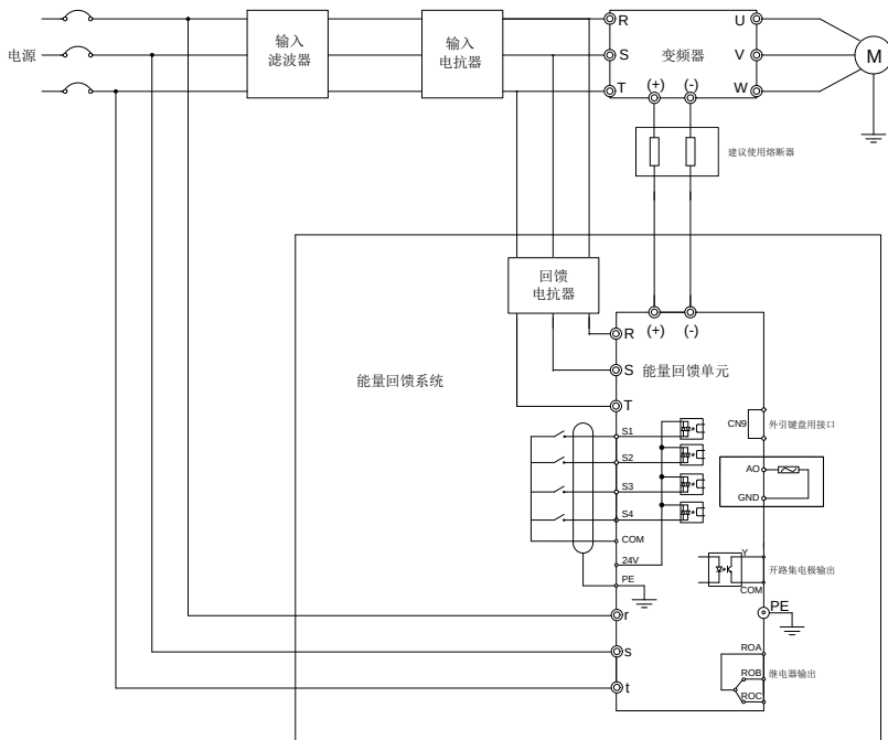
图 4-6 380V 55kW~250kW 及 660V 55kW~400kW 标准接线
