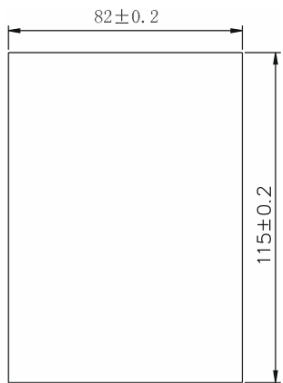
图 9-2 外引键盘（大）的开孔尺寸
