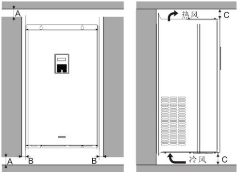
图 4-1 安装距离
