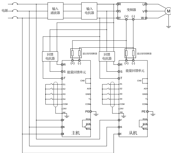
图 4-7 RBU100H 并机接线 1
