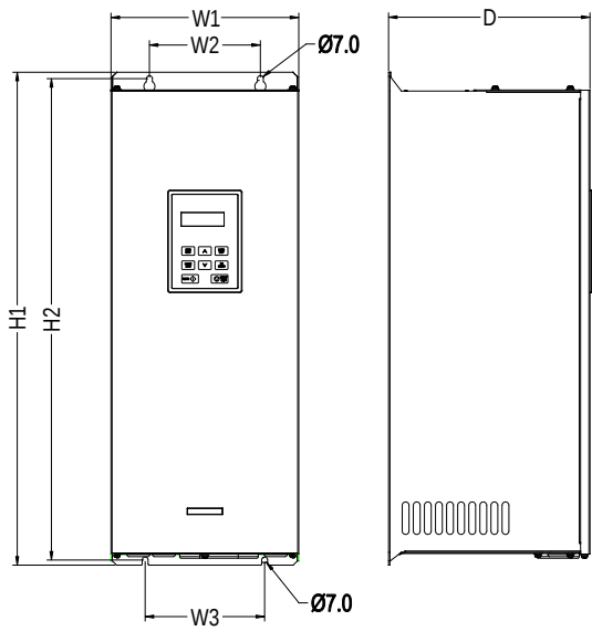
图 9-3 壁挂式能量回馈单元外形尺寸及安装尺寸
