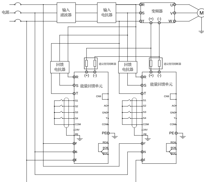
图 4-8 RBU100H 并机接线 2
