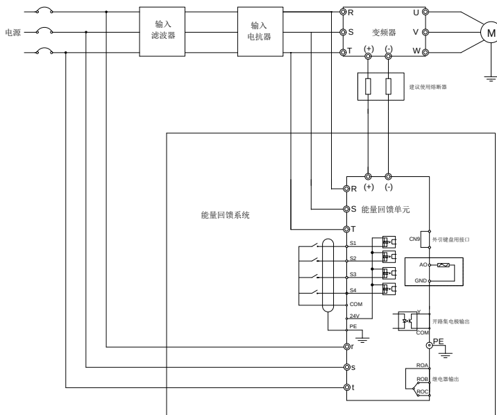
图 4-5 380V 22kW~45kW 标准接线
