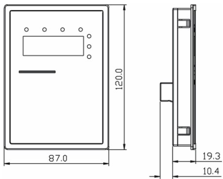
图 9-1 外引键盘（大）的安装尺寸
