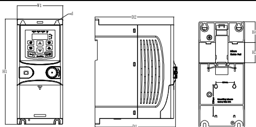
图 D-2 导轨安装
