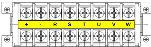
图 C-5 2.2kW 以下-4 机型接线端子
