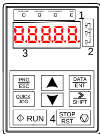
图 4-2 4kW（含）以上机型键盘示意图
