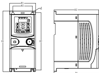
图 D-1 壁挂安装
