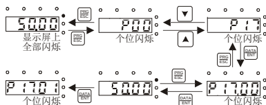
图 4-6 查看参数示意图
