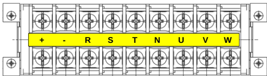
图 C-4 4~37kW 接线端子
