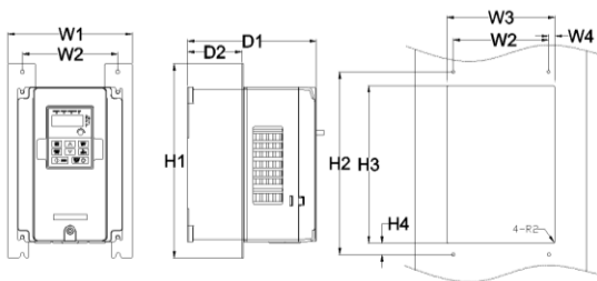
图 D-4 法兰安装
