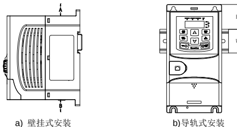
a) 壁挂式安装
