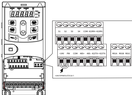
图 3-3 2.2kW 及以下 U 型短接位置示意图
