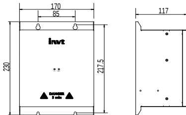
图 A-2 升压模块安装尺寸图
