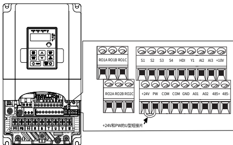
图 3-4 4kW 及以上 U 型短接位置示意图
