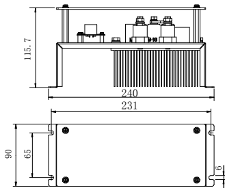
图 C-2 切换模块安装尺寸 (单位: mm)
