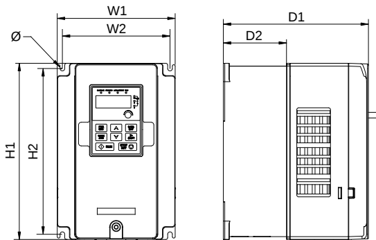
图 D-3 壁挂安装
