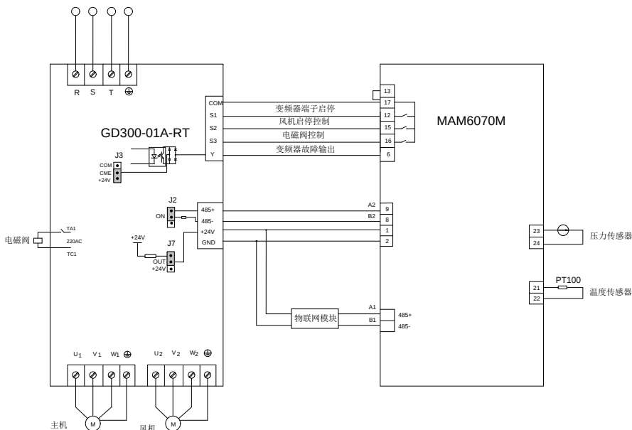
图 4-13 普乐特控制器 6070M+GD300-01A-RT 变频器接线
