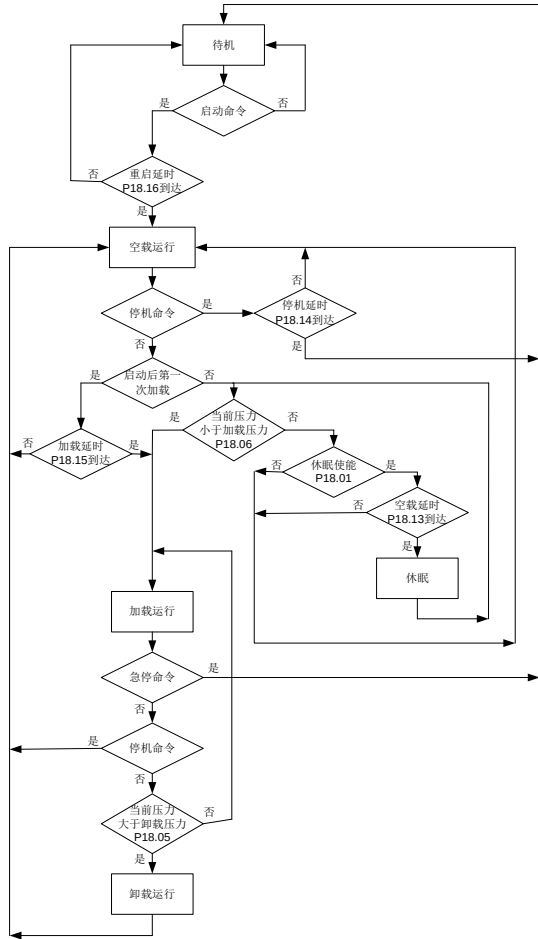
图 5-1 空压机控制逻辑
