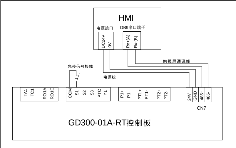
图 C-1 触摸屏标配线缆连接
