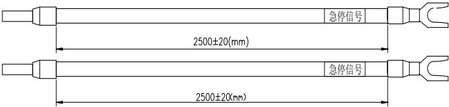
图 C-2 急停线示意图
