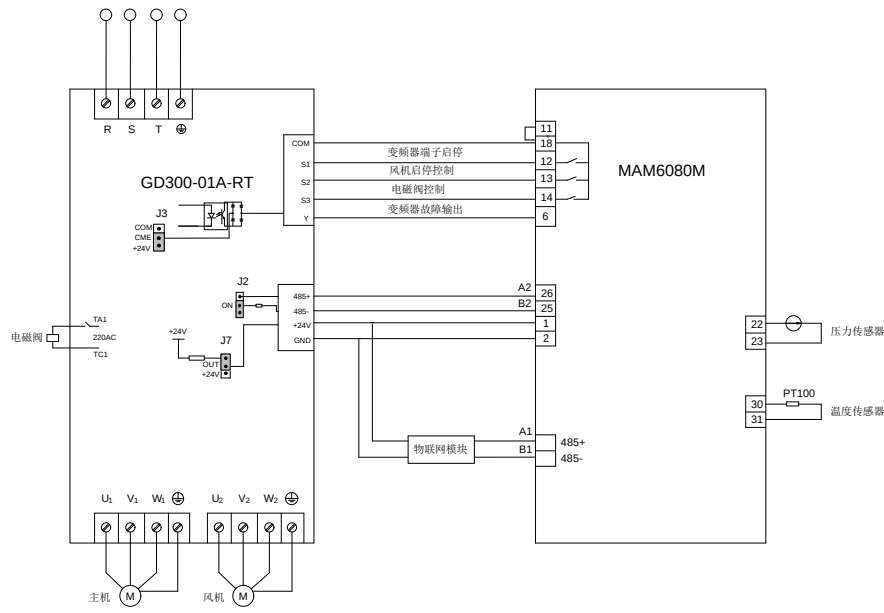
图 4-14 普乐特控制器 6080M+GD300-01A-RT 变频器接线
