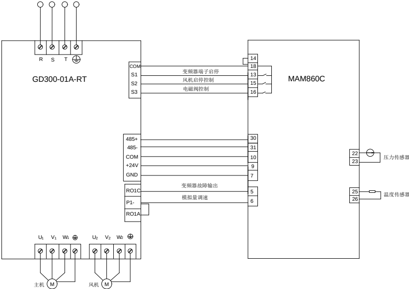
图 4-22 系统接线
