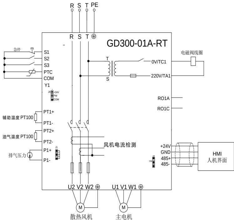
图 4-1 HMI+GD300-01A-RT 变频器接线
