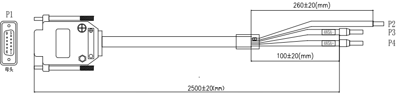
图 C-4 触摸屏通讯线示意图
