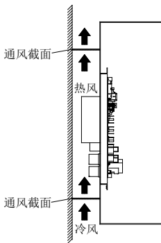
图 4-4 通风截面
