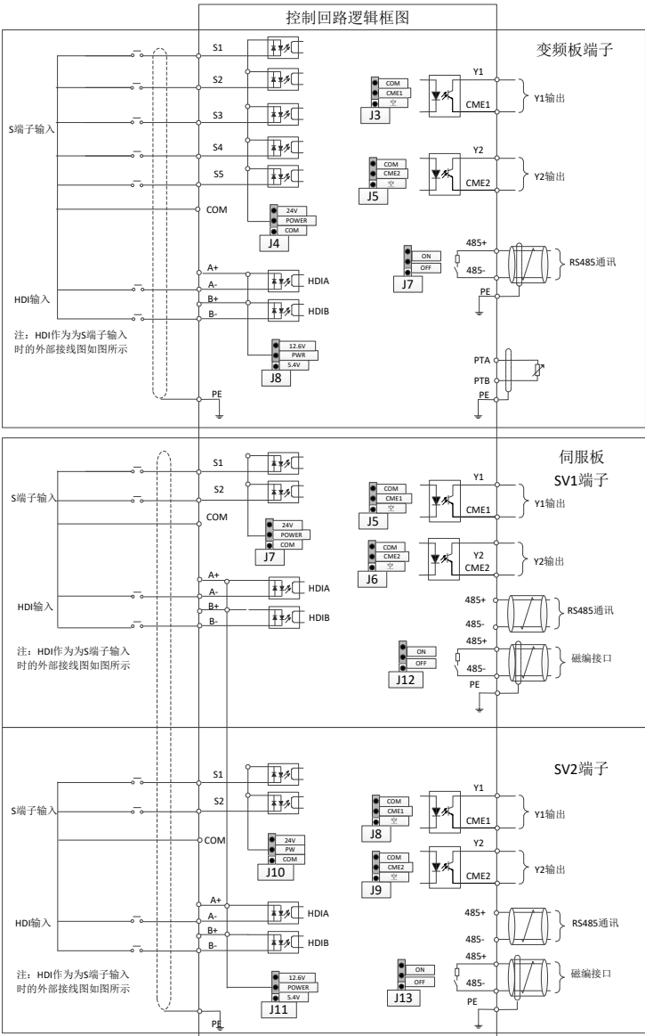
图 4-8 控制回路接线
