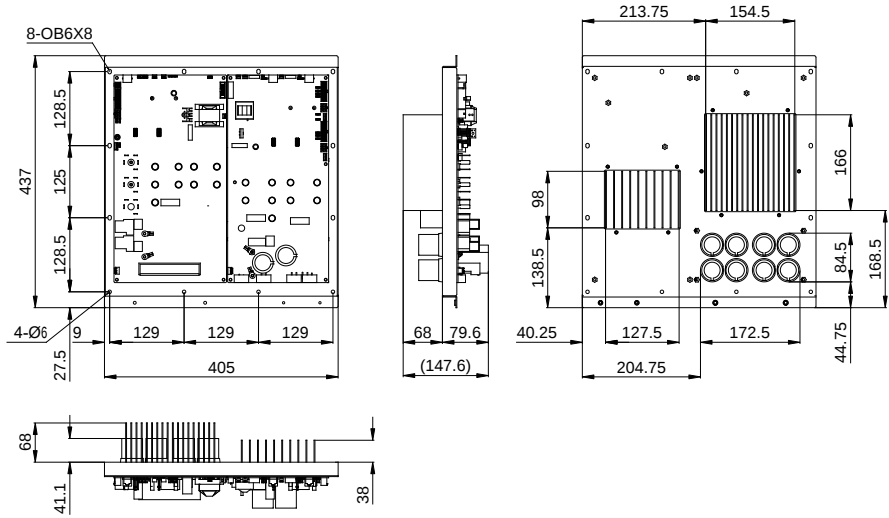
图 C-4 三合一安装尺寸
