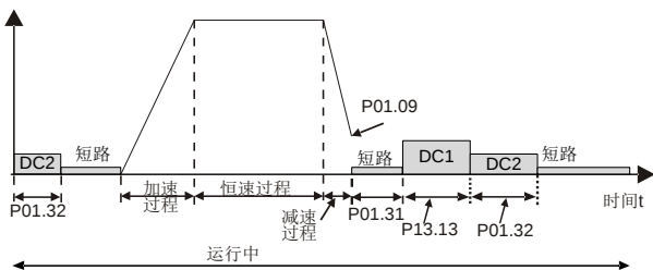
图 6-1 启停制动示意图
