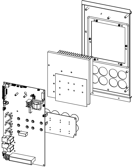
图 C-3 单变频结构
