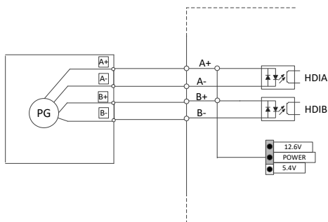
图 4-10 与差分型编码器配套使用时的外部接线
