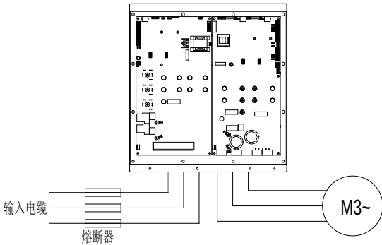
图 4-12 熔断器配置
