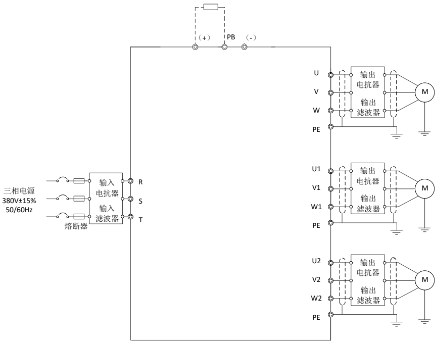
图 4-5 主回路接线
