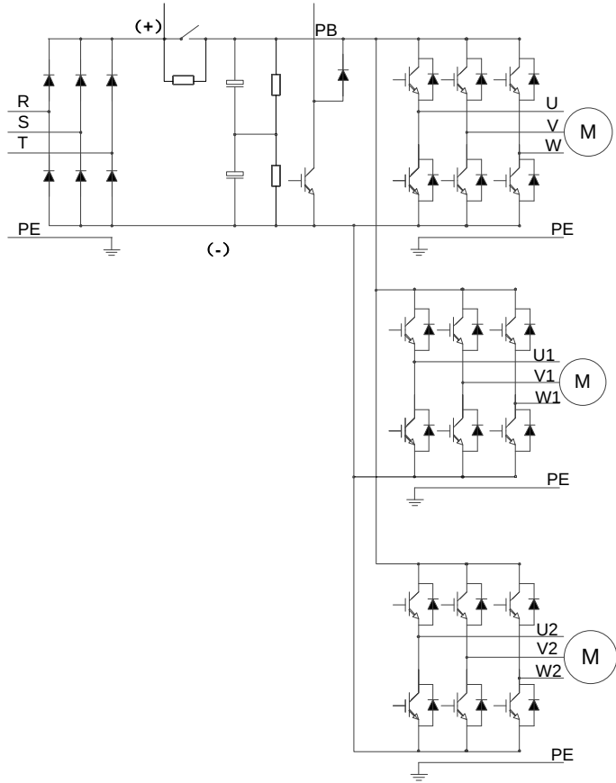
图 3-1 主回路简图
