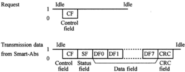
图 11-6 磁编通讯格式
