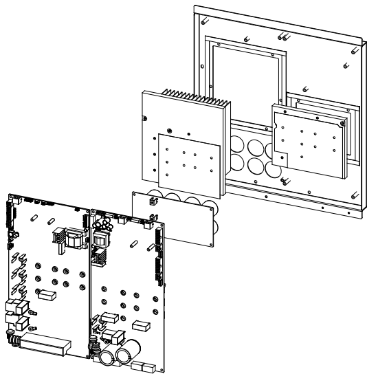
图 C-2 三合一结构
