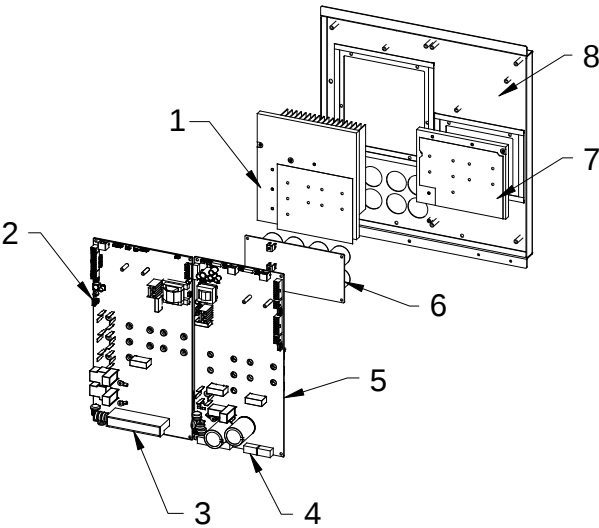
图 3-3 产品结构
