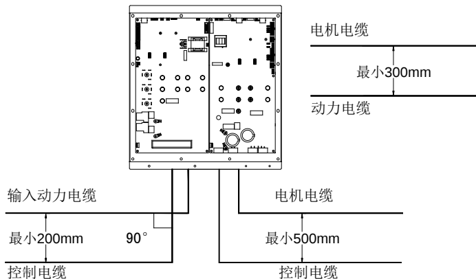
图 D-3 布线距离
