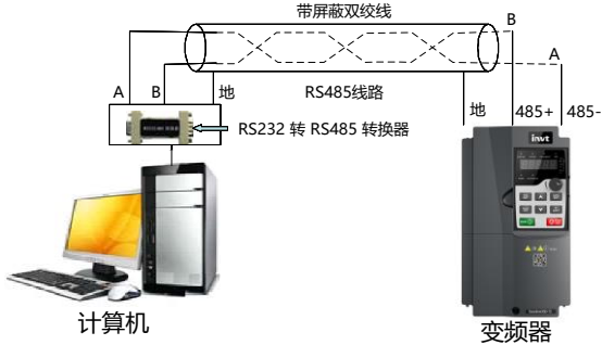
图 11-1 RS485 单机应用时的物理接线图
