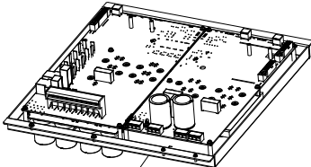
钣金支架需接地导通
