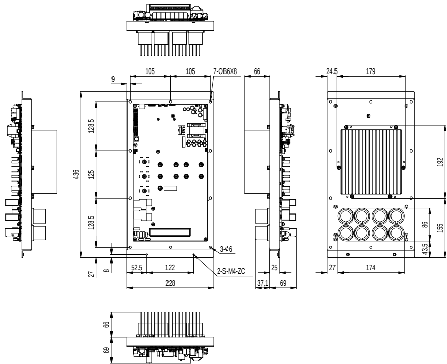
图 C-5 单变频安装尺寸
