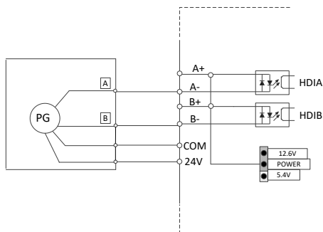
图 4-9 HDI 与推挽型编码器配套使用时的外部接线
