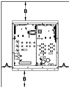
图 4-3 单台安装
