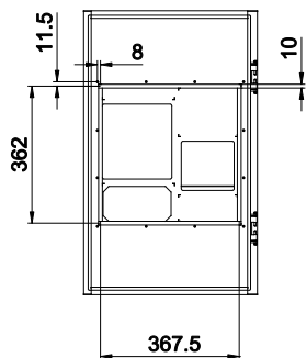
防水胶条推荐尺寸
