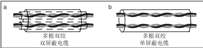
图 D-2 动力电缆布线
