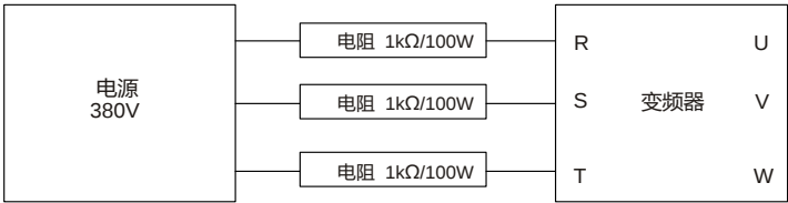
图 10-1 380V 驱动装置充电电路示例
