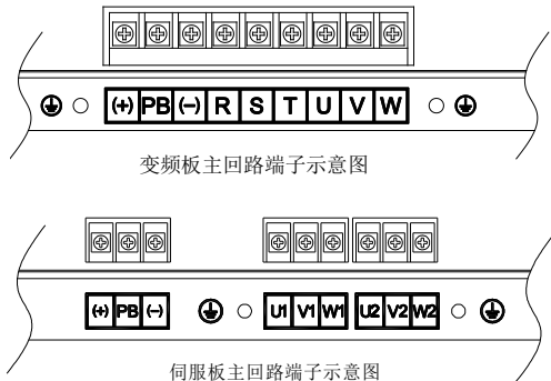
图 4-6 主回路端子
