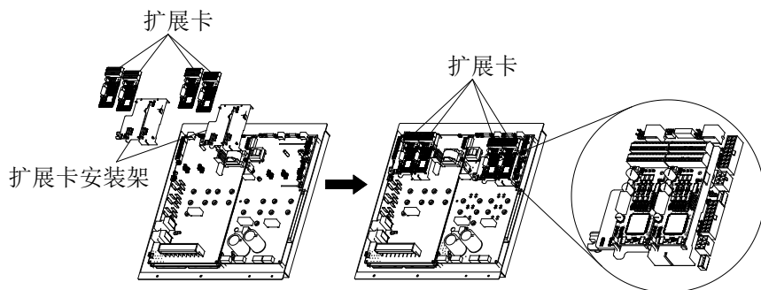
图 A-1 扩展卡安装效果
