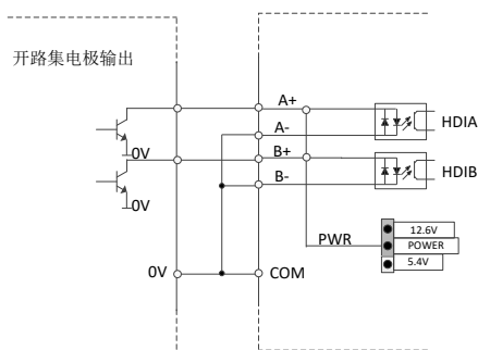
图 4-11 与集电极开路编码器配套使用时的外部接线
